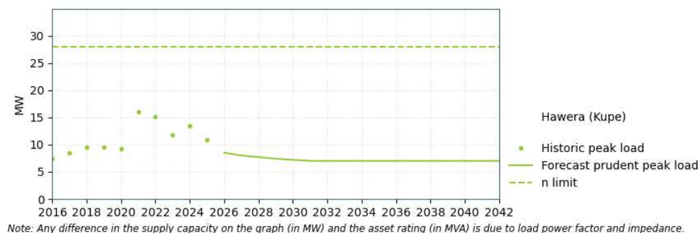
Figure 12-6: Hawera (Kupe) supply capacity
